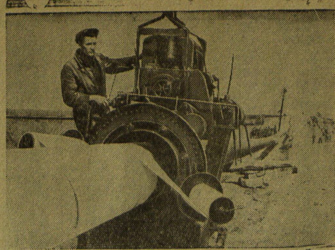
ЛЕНИНГРАДСКАЯ ОБЛАСТЬ. На строительстве газопровода Кохтла-Ярве—Ленинград. На снимке: изоляция сварных труб газопровода специальной машиной. За работой машиниста-стахановец Н. В. Новиков.
